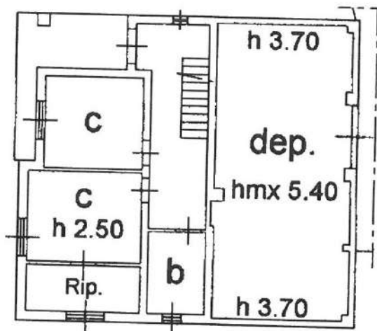
Piano primo
